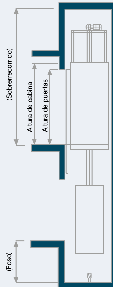
SECCIÓN VERTICAL
