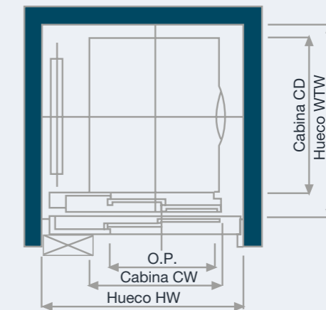
CROQUIS DE PLANTA
